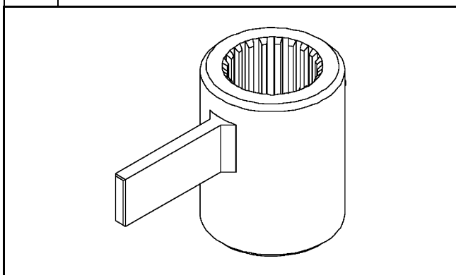
Attrezzatura per rilievo gioco. CA715146
